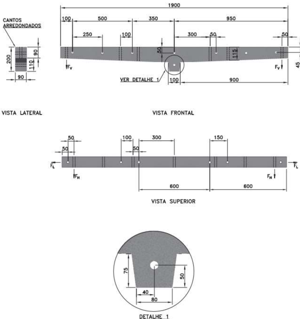
Figura 2 - Cruzeta de concreto armado normal para rede compacta com furação extra - tipo "T"- 1900 mm
