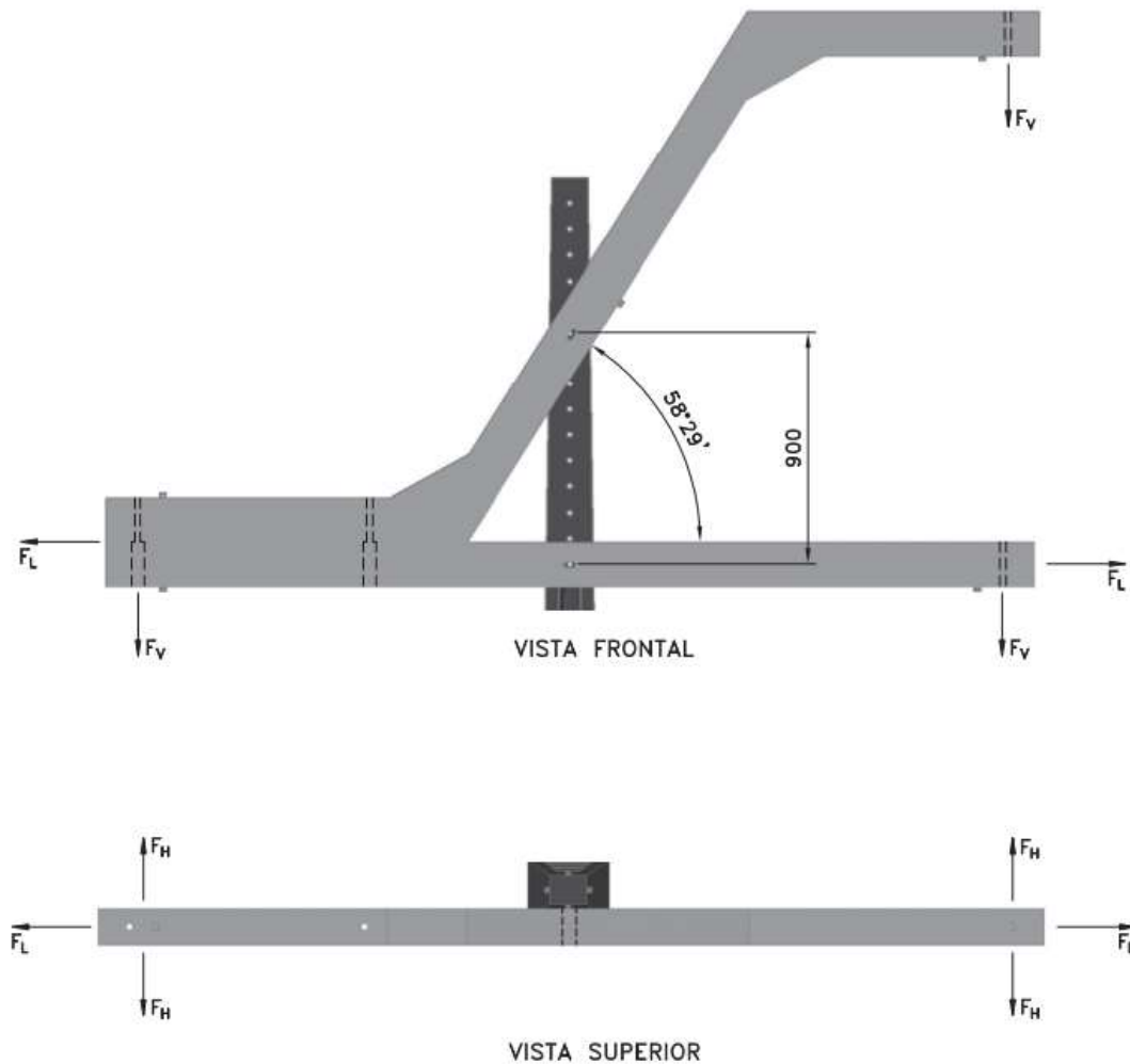
Figura 22 - Cruzetas de concreto armado - Tipo "Z" e "I" esforços
