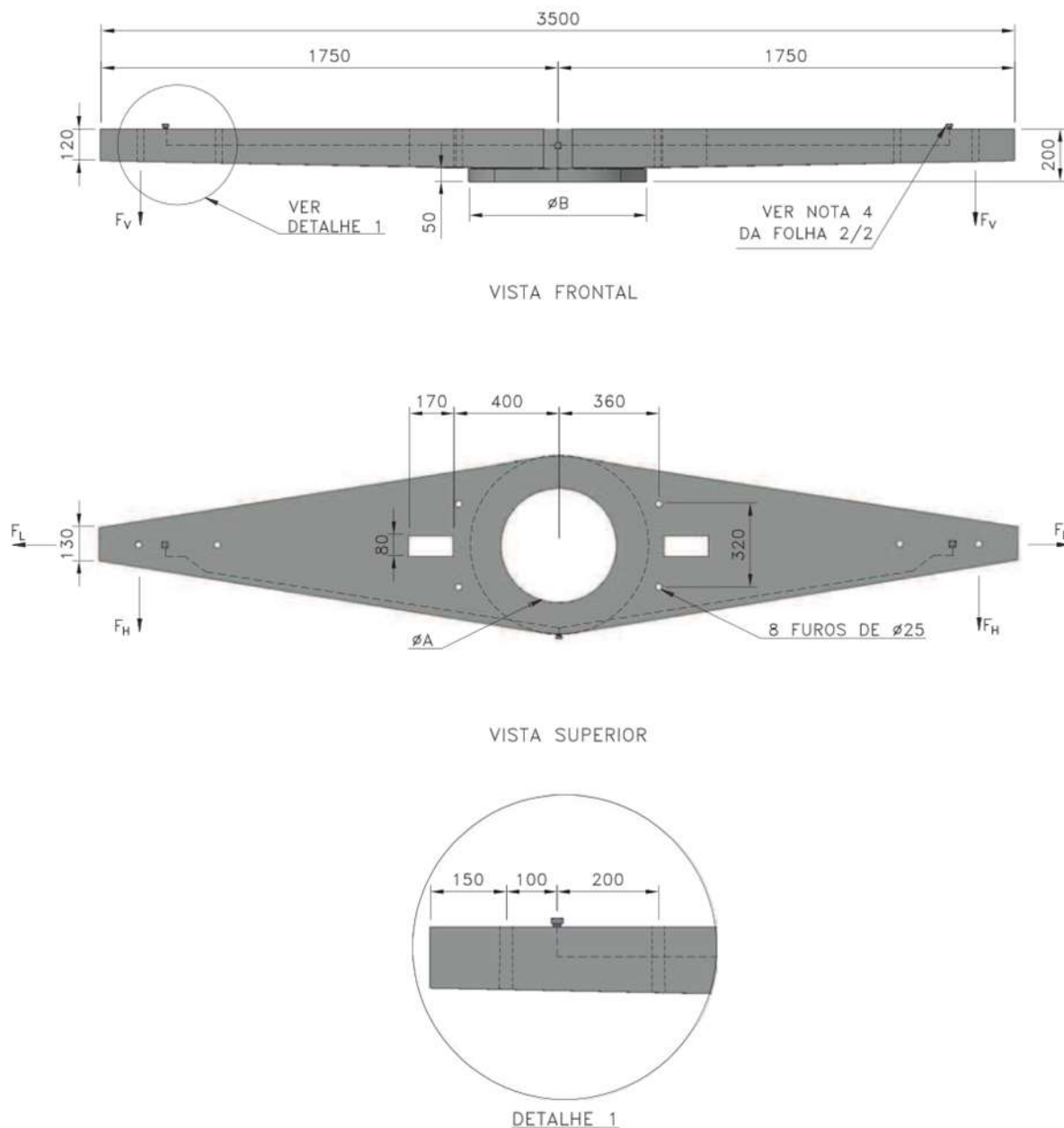
Figura 13 - Cruzeta de concreto armado modelo simples – 3500mm
