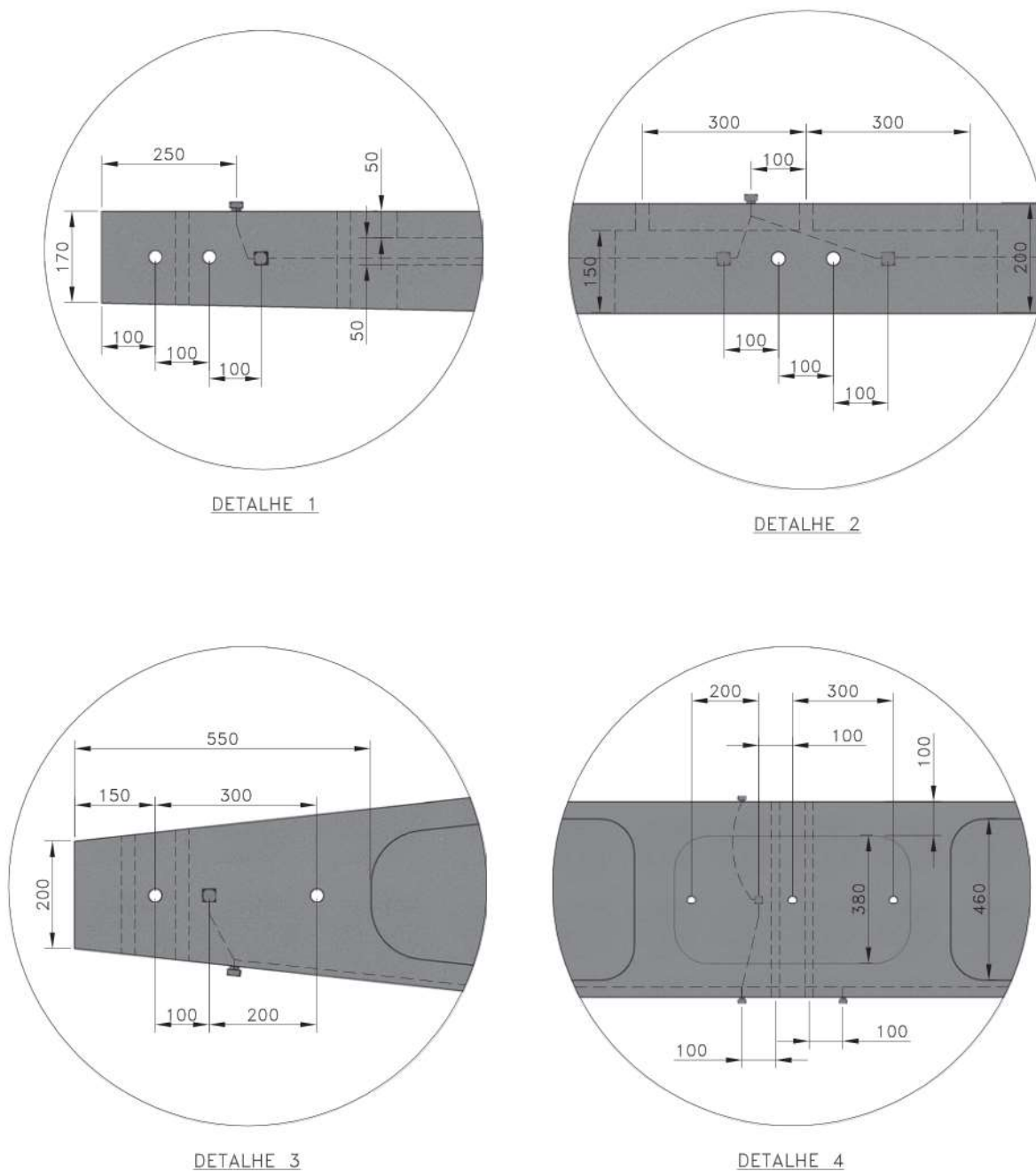
Figura 19 - Cruzeta de concreto armado dupla - tipo "H" – 9200mm
