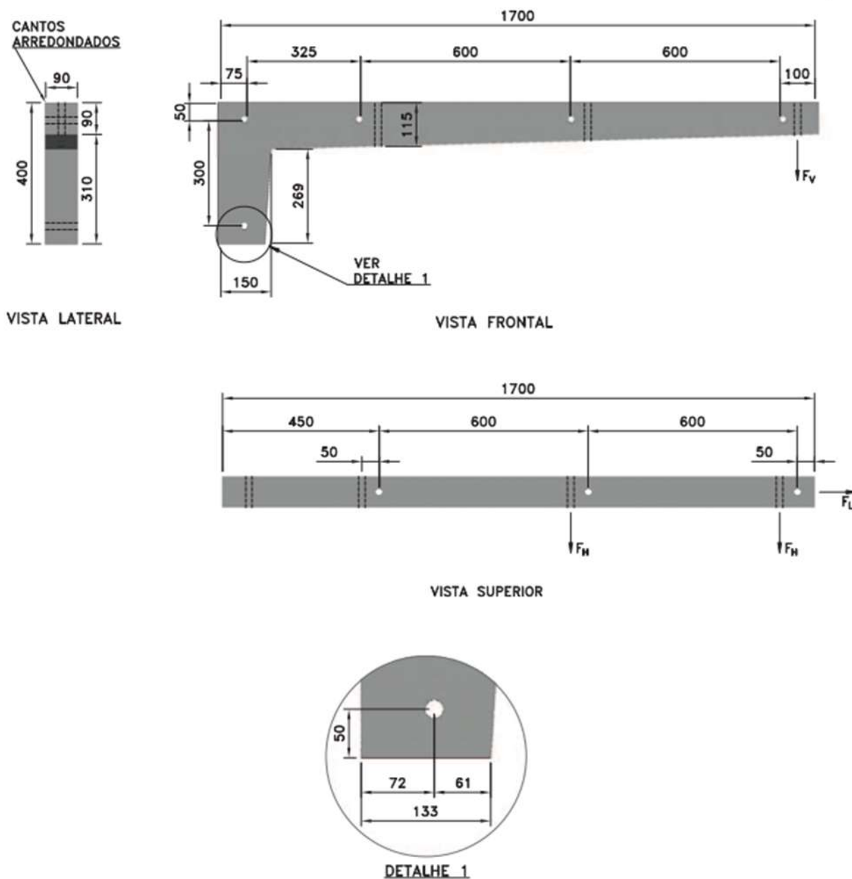
Figura 6 - Cruzeta de concreto armado - tipo "L" – 1700mm
