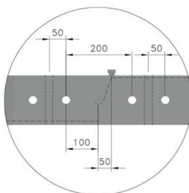
DETALHE 1
