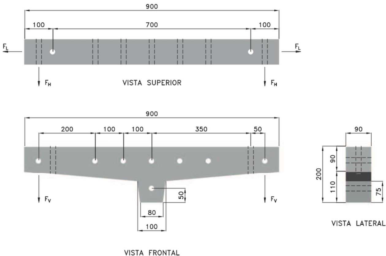
Figura 3 - Cruzeta de concreto armado normal para rede compacta - tipo "T" - 900mm
