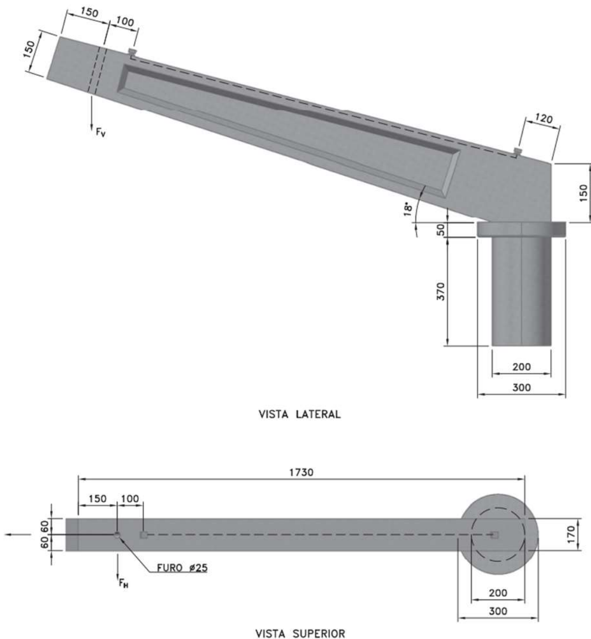
Figura 20 - Cruzeta de concreto armado pivotante
