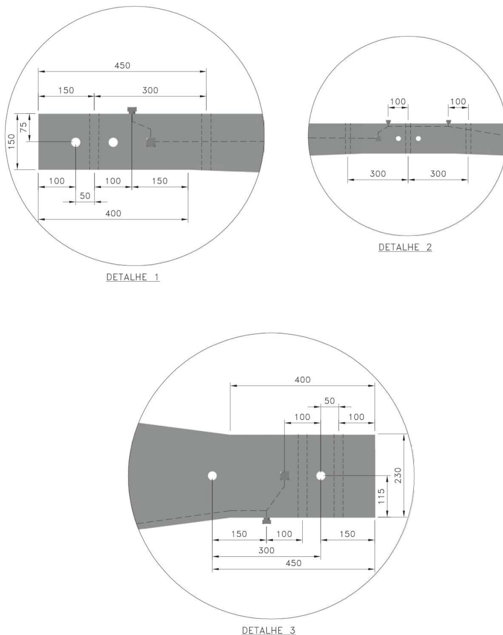
Figura 16 - Cruzeta de concreto armado simples - tipo "H" – 6700mm – detalhes
