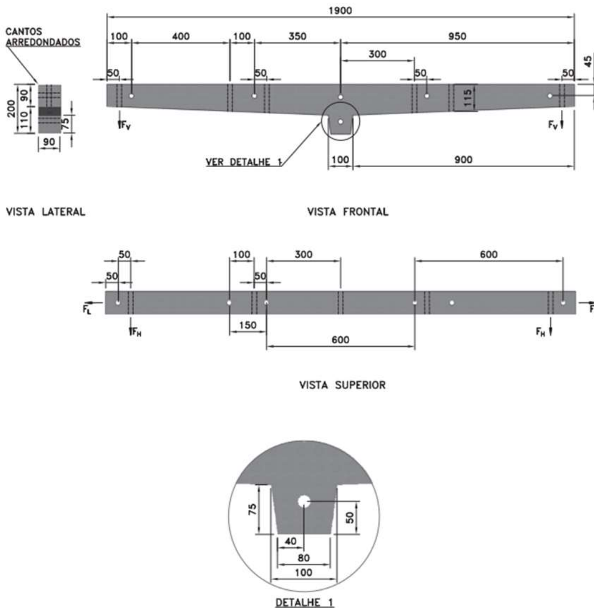
Figura 1 - Cruzeta de concreto armado normal – Tipo “T” – 1900mm
