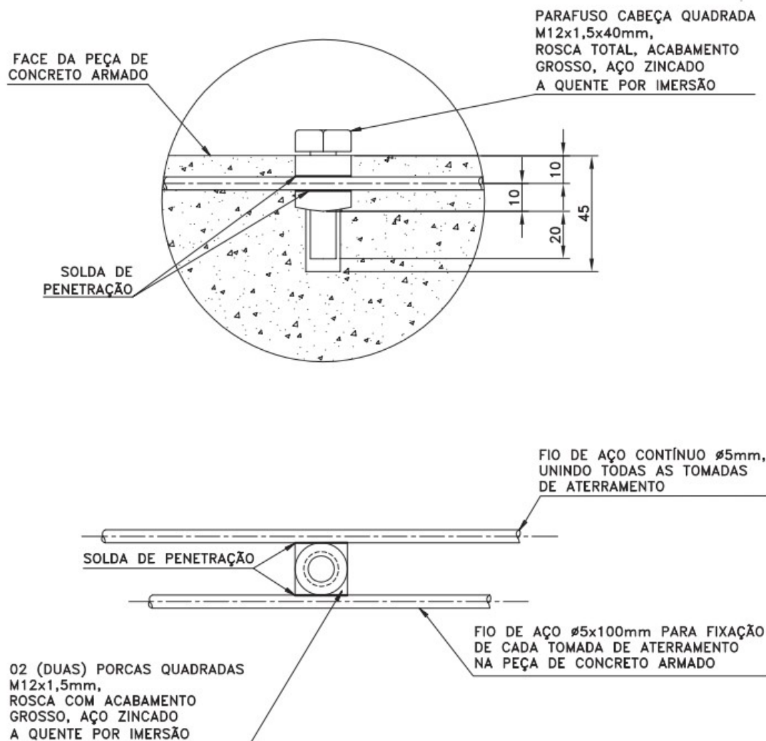
Figura 23 - Tomada de aterramento
