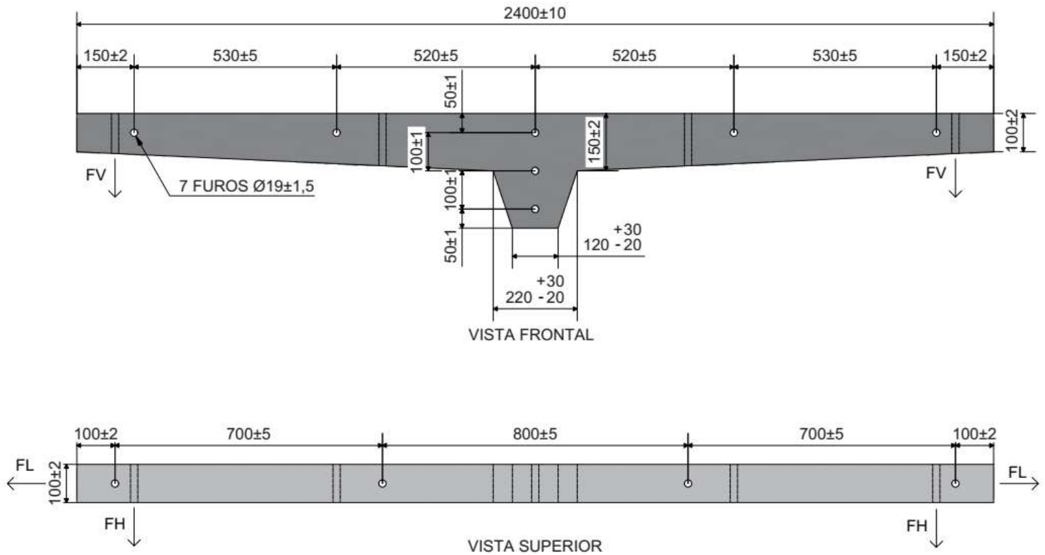
Figura 10 - Cruzeta tipo T de 2 400 mm com 500 daN
