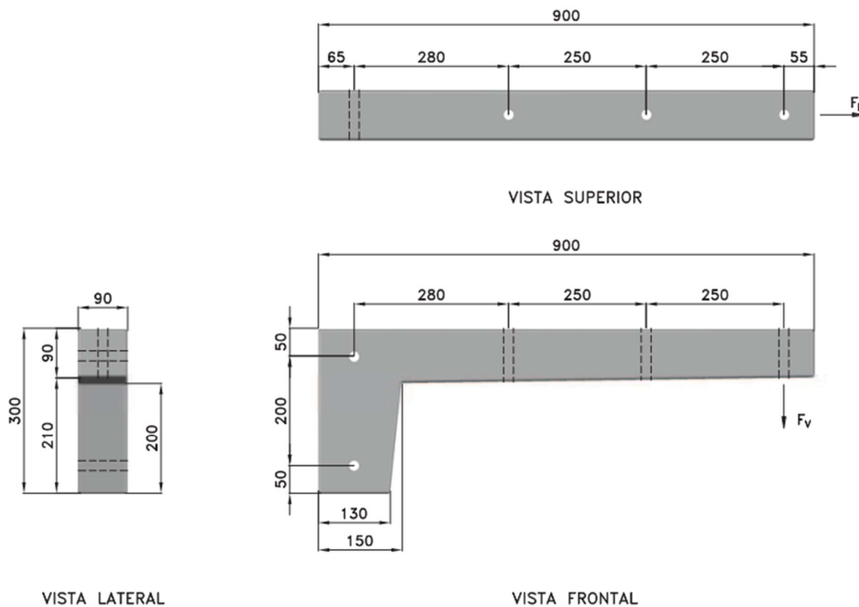
Figura 7 - Cruzeta de concreto armado meio beco para rede compacta – 900mm
