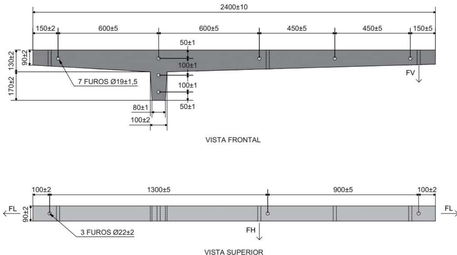
Figura 12 - Cruzeta MB 2 400 mm com 300 daN
