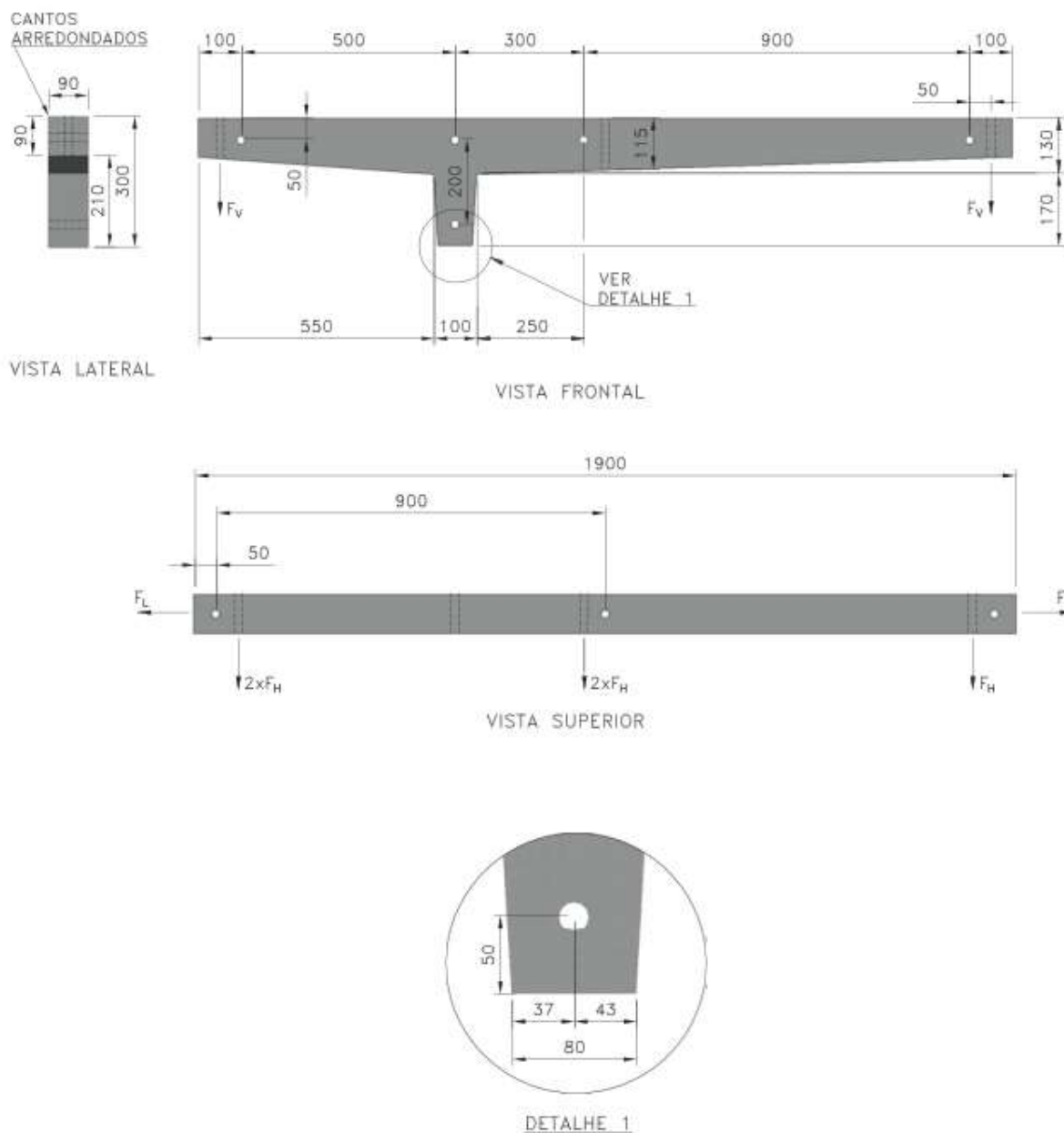
Figura 5 - Cruzeta de concreto armado meio bico - tipo "MB" – 1900mm
