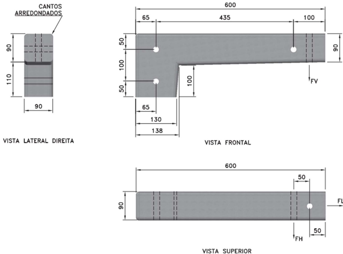
Figura 8 - Cruzeta de concreto armado para MRT - tipo "L" – 600m
